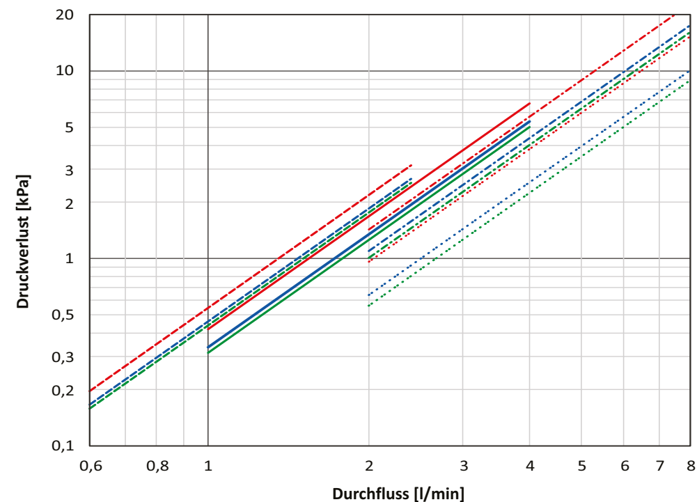
Druckverlustdiagramm Verteiler
