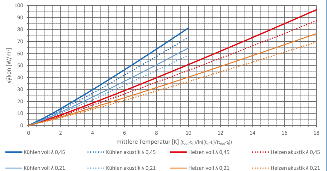
Delgado auf GKP gelegt Heiz- und Kühlleistung
