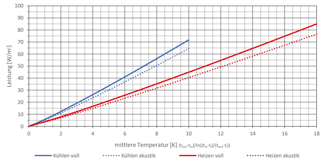
Aktive Gipskartonplatten Heiz- und Kühlleistung
