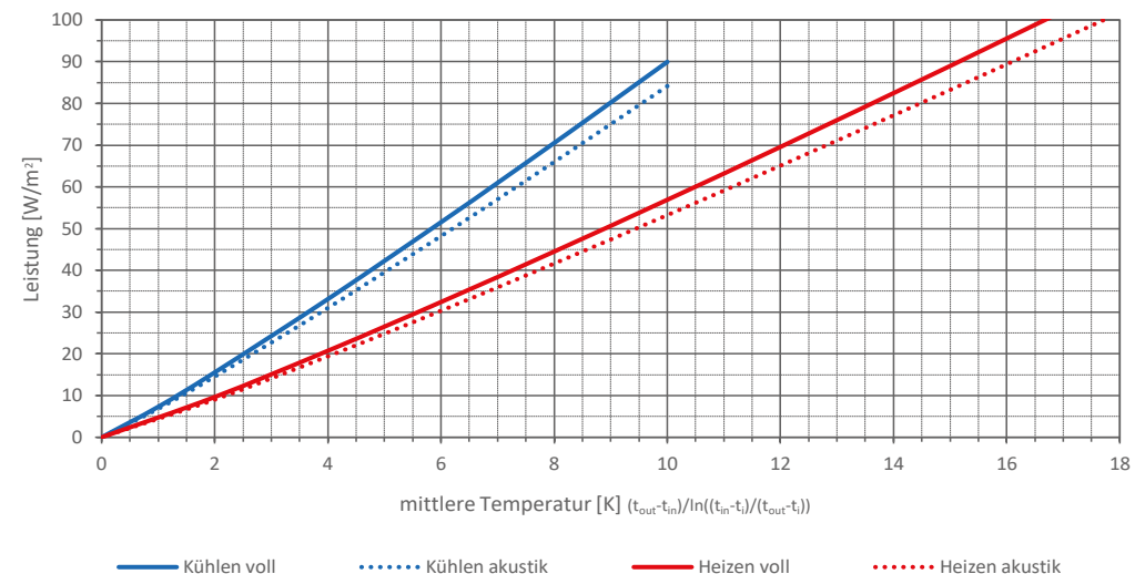
Delgado im Metallkassette Heiz- und Kühlleistung
