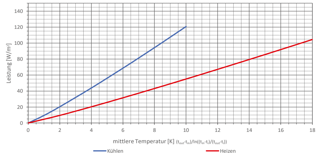
Delgado Profil 40x30 Heiz- und Kühlleistung
